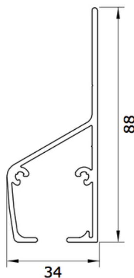
Geleider voor montage zijkant ligger
