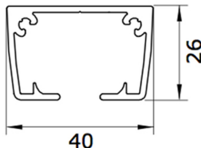
Geleider voor montage onder de ligger
